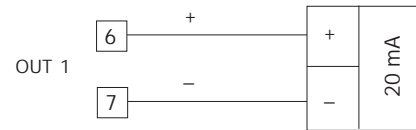
Abb.10 ANSCHLUSS mA-AUSGANG Dieser Ausgang ist isoliert. Die Höchstbelastung beträgt 500 Ω.
